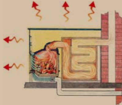
Speicherofen, Wärmeabgabe über Wärmestrahlung.
